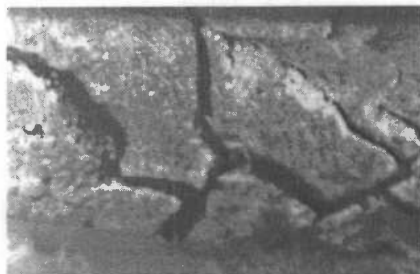
Сл. 8 – Јамице и пукотине присутне на микрографији наменских испуна од кермет глас-јономер цемента у пределу водећих површина (SEM 3000 ×).
