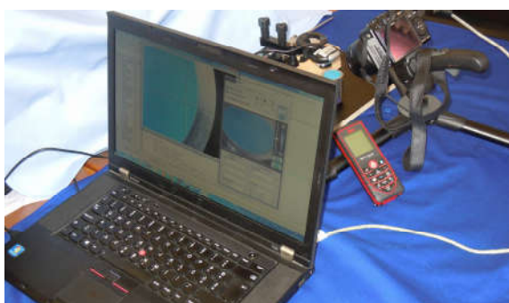
Slika 6.14. Eksperimentalna postavka
